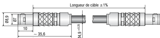
SC6000-1,0 Câble de synchronisation (N° art. 2903473)
