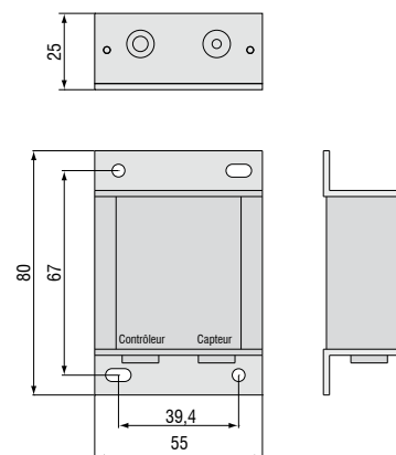
Préamplificateur capacitif CP6001
