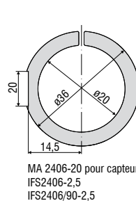
Bague de montage
