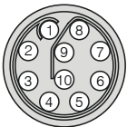
Connecteur de câble 10 pôles Vue côté brasage
