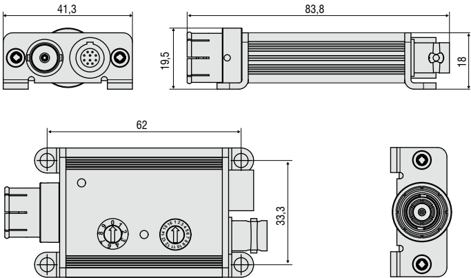
Dimensions en mm (non à l'échelle)
