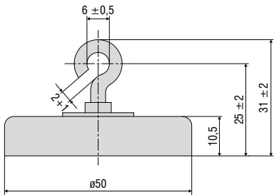
MH1-WDS Support magnétique pour fixation du câble
