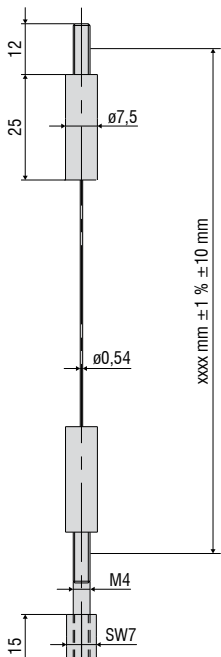
WE-xxxx-M4 Rallonge de câble avec raccord M4, x=longueur de câble
