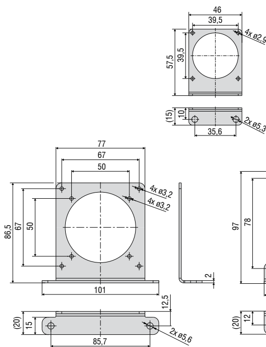
WPS-MB77 pour la série MK77
