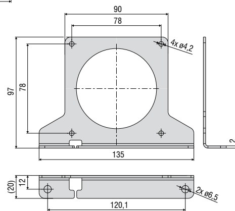
WPS-MB88 pour la série MK88
