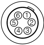
Vue côté soudure, connecteur femelle 6 points
