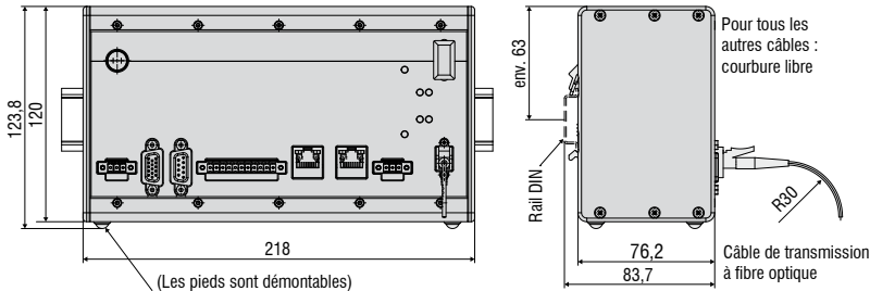
Contrôleur IFC2421
