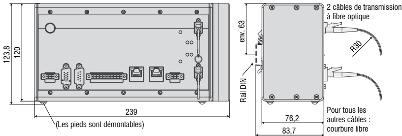
Contrôleur IFC2422
