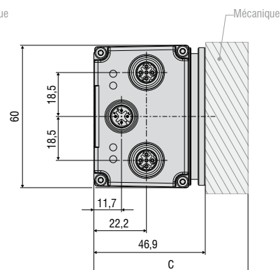
Sortie PN/ENIP/CAT
