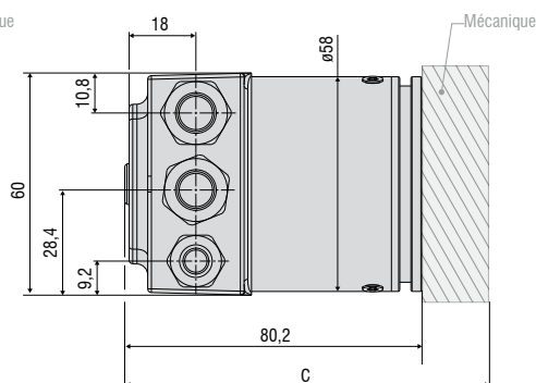
Sortie CO/PB
