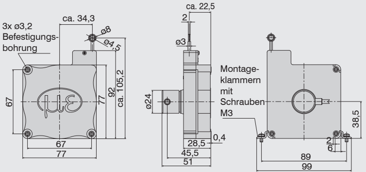
Maßzeichnung WPS-2100-MK77 mit Inkrementalencoder, Abmessungen in mm
