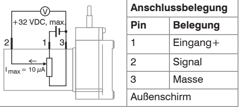
Anschlussbelegung WPS-2100-MK77 mit Potentiometerausgang
