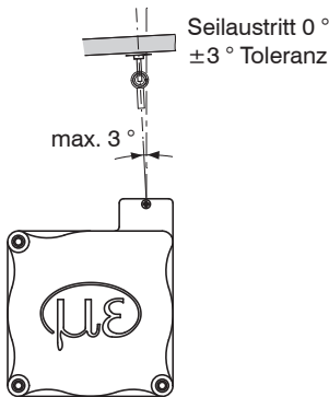
Befestigung und maximaler Schrägzug des Messseils
