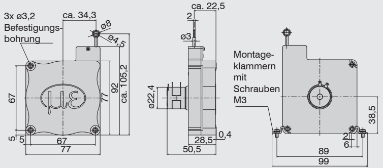
Maßzeichnung WPS-2100-MK77 mit Potentiometer, Abmessungen in mm
