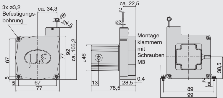
Maßzeichnung WPS-2100-MK77 mit Potentiometer und integriertem Kabel, Abmessungen in mm
